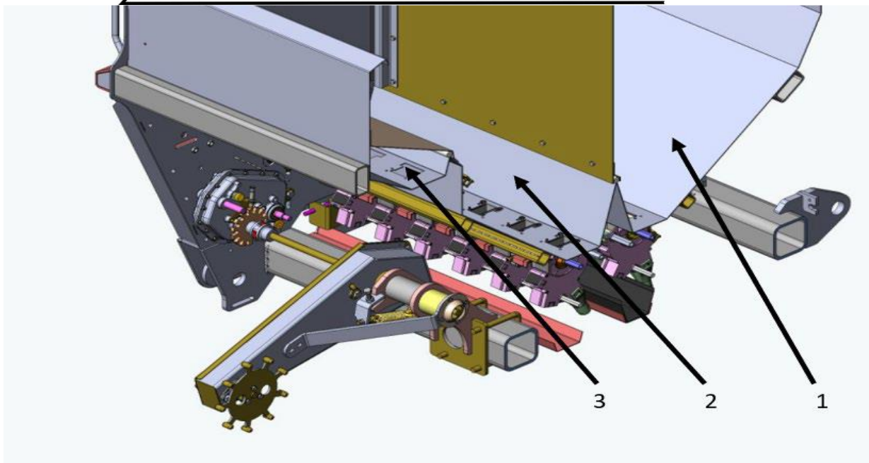
Obrázek 2) Průřez CEREX EVO, 1.zásobník hnojiva, 2 zásobník osiva, 3 zásobník na malá semena (option)
